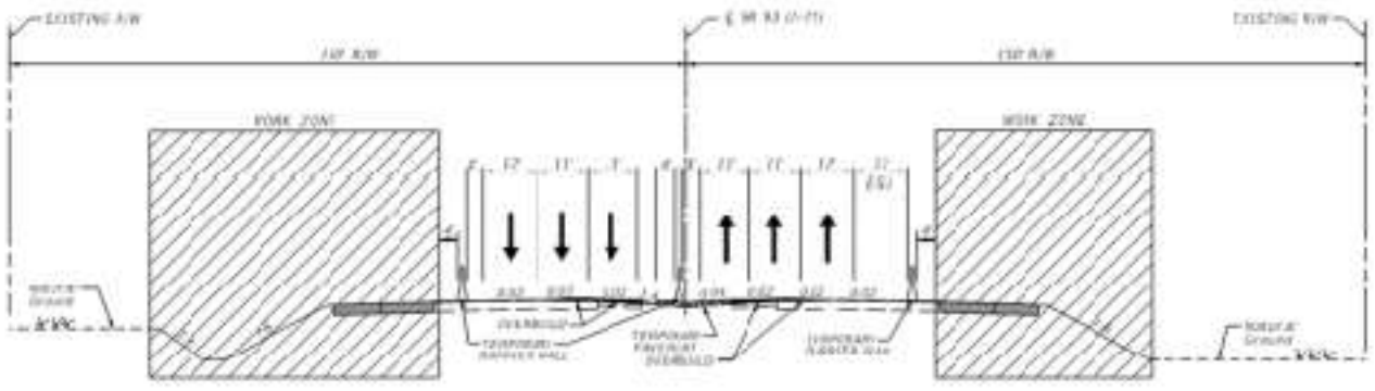
SR 93 (I-75) STA. 2388+00.00 TO STA. 2440+80.00 PHASE 2
